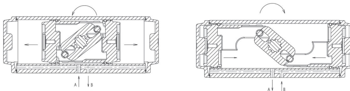
Двустороннего действия
