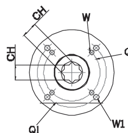
ПРИСОЕДИНЕНИЕ АРМАТУРЫ
